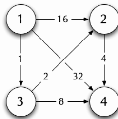
Figur 1: Grafen G = (V, E)
